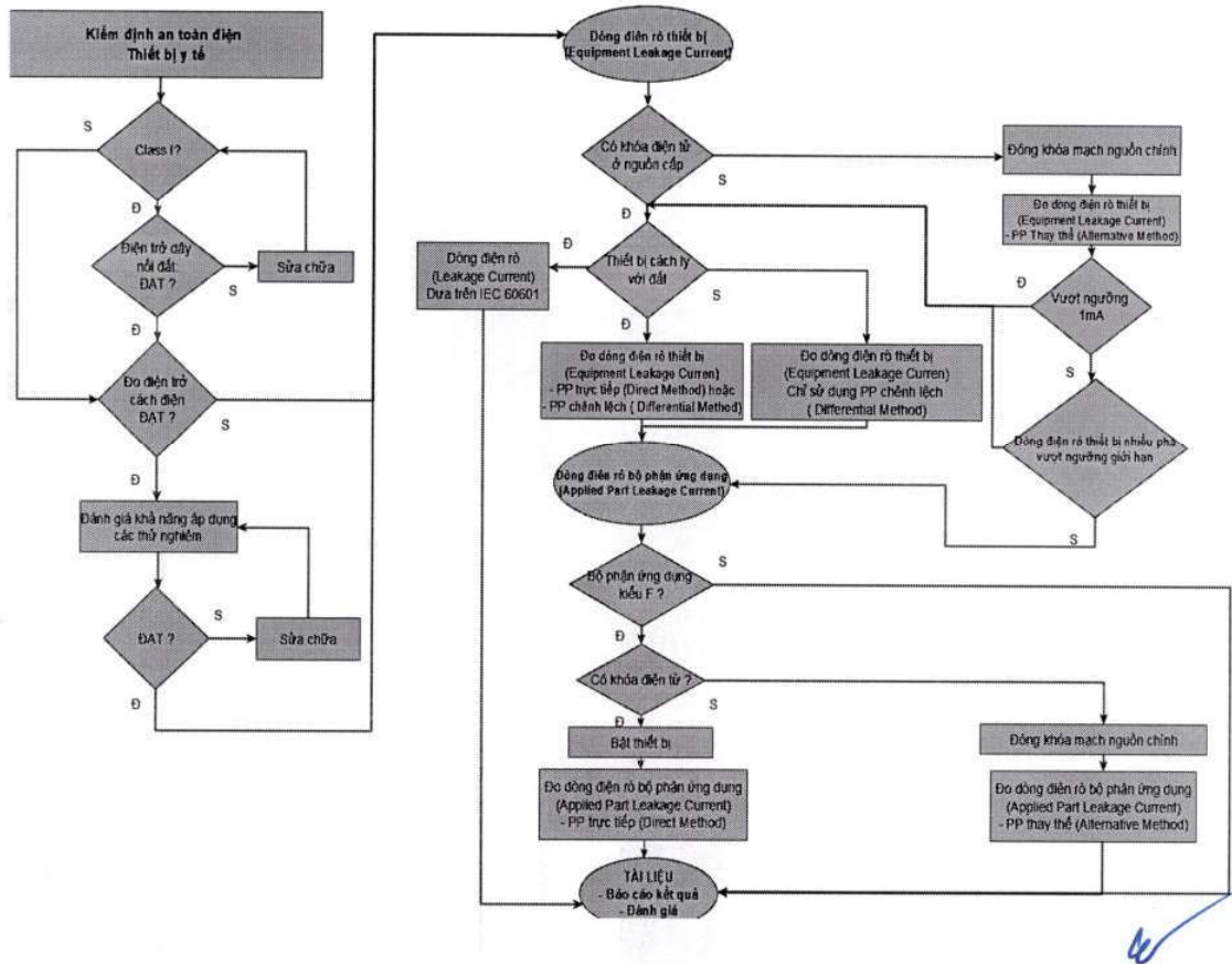
Hình 6. Lưu đồ đo dòng điện rò
