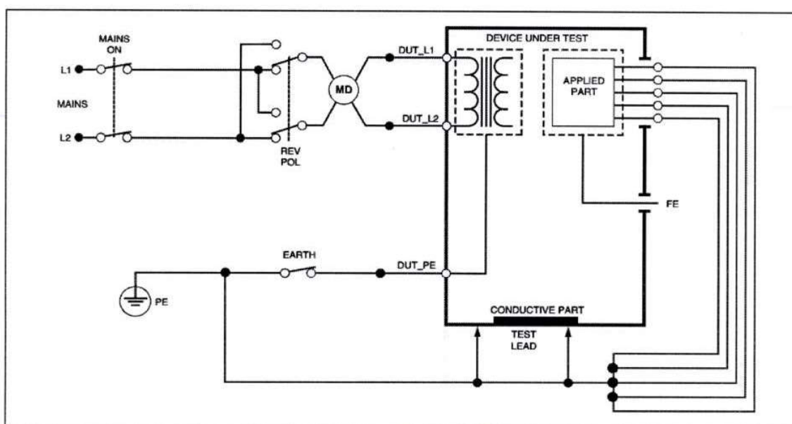
Hình 8. Phương pháp đo dòng điện rò qua thiết bị bằng phương pháp chênh lệch
