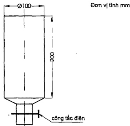
Hình 1 – Kích thước và kết cấu vách ngăn lấy bột
